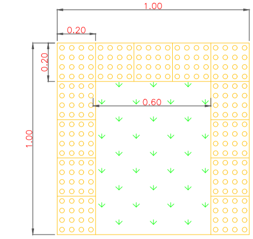
Detalhe 1 - Canteiro árvores Esc 1:20
