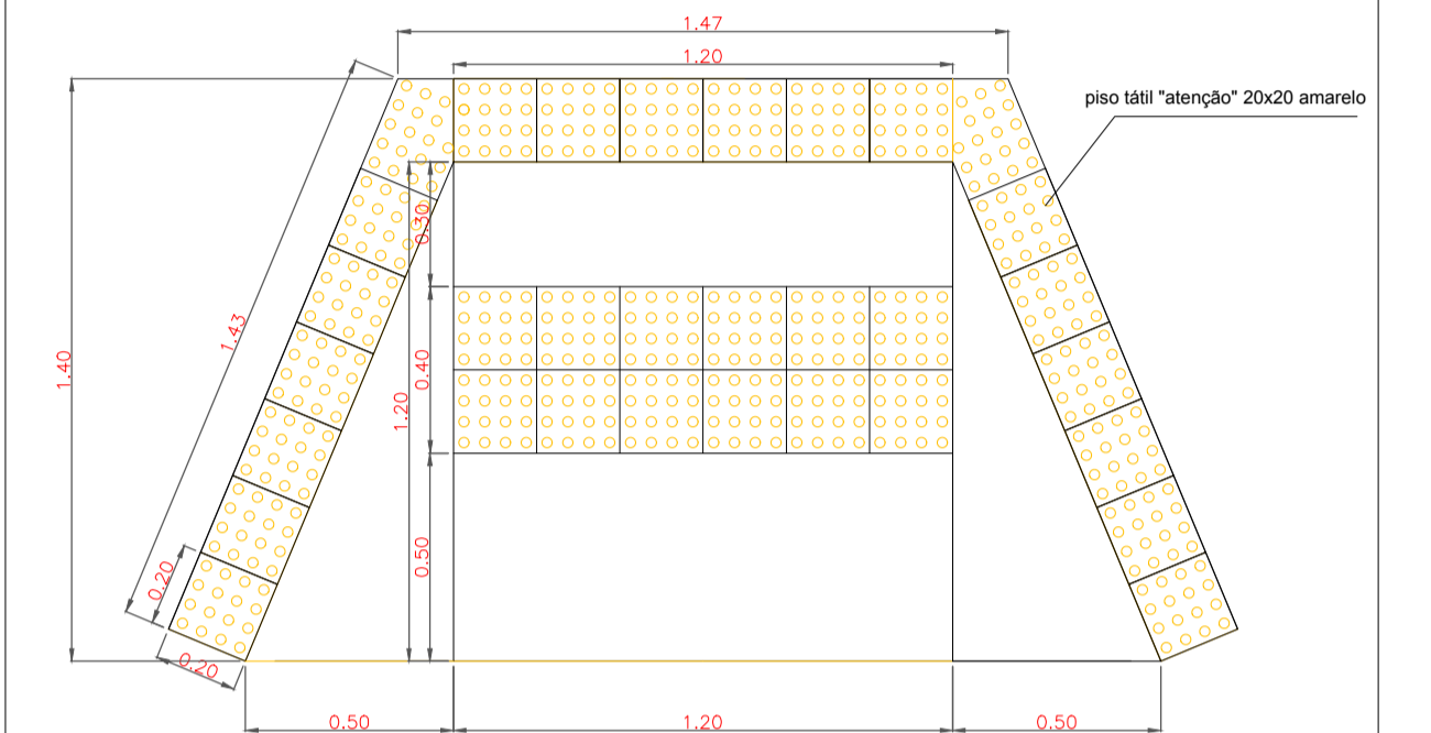
Detalhe 2 - Rampa acesso PNE Esc 1:20
